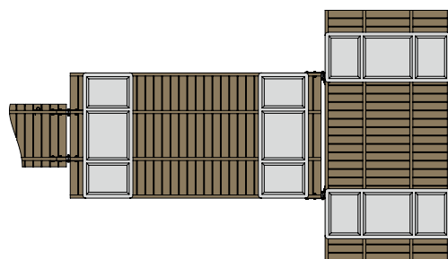
T-CONNECTION
